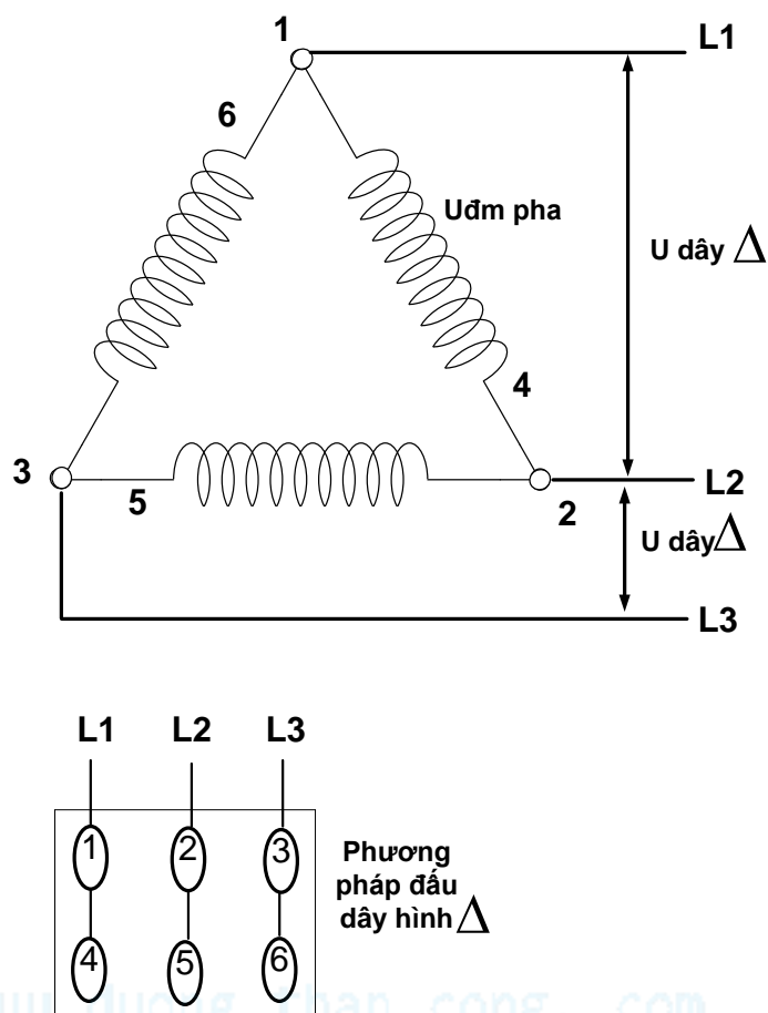
Hình 1.8 : Sơ đồ đấu dây quấn stator theo hình \Delta .
